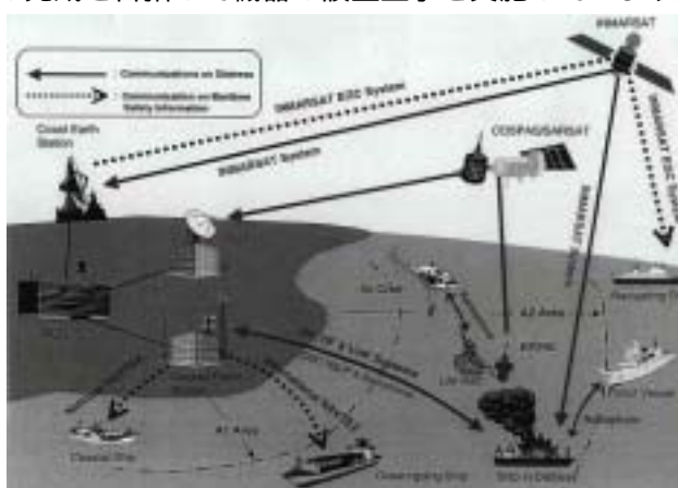
GMDSS 概念図
